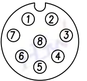
HGF01.5-M808P-CB
