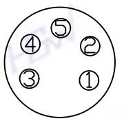
HGF02-M805'P-CB
